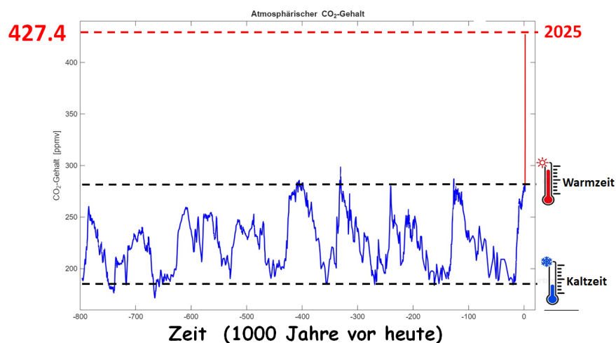
Abb. 2: Zeitliche Entwicklung des CO 2 -Gehalts der Luft seit 800.000 Jahren, ermittelt aus Lufteinschlüssen im EPICA Dome C (Antarktis) Eiskern (blau, Lüthi, D. et al., 2008) und direkten Messungen von Luftproben auf Mauna Loa (seit 1959, rot, Datenquelle: https://gml.noaa.gov/ccgg/trends/data.html ).
