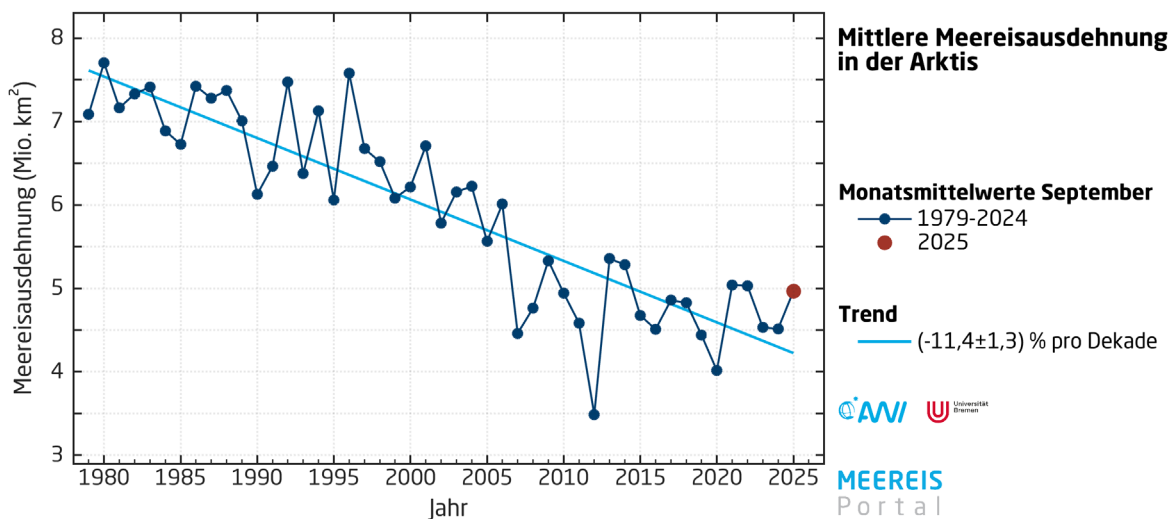
Abb. 6: Rückgang der sommerlichen Meereisausdehnung in der Arktis (Grafik: meereisportal.de).
