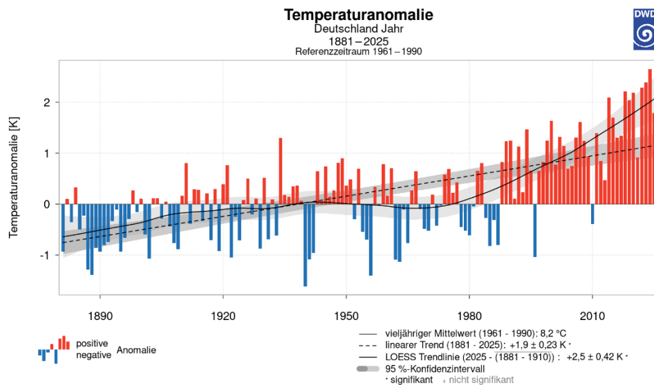
Abb. 5: Entwicklung der Temperaturanomalien in Deutschland von 1881 – 2025 (Grafik: Deutscher Wetterdienst).
