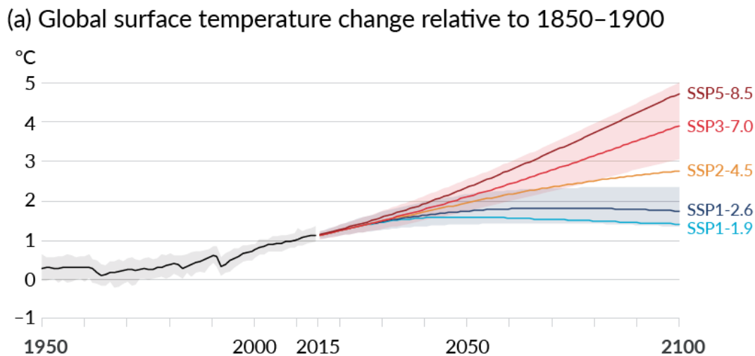
Abb. 8: Anstieg der globalen Oberflächentemperatur bis zum Ende dieses Jahrhunderts für verschiedene Energieszenarien (IPCC AR6 (SPM), Fig. SPM.8) (Grafik: https://www.ipcc.ch/report/ar6/wg1/ ). Die Schattierungen geben die entsprechenden Unsicherheitsbereiche an.
