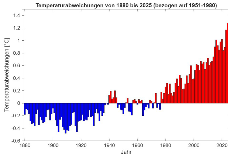
Abb. 4: Global gemittelte Anomalien der Lufttemperatur an der Erdoberfläche. (Abweichungen vom Mittelwert der Jahre 1951-1980; Datenquelle: GISS, http://data.giss.nasa.gov/gistemp/ ).
