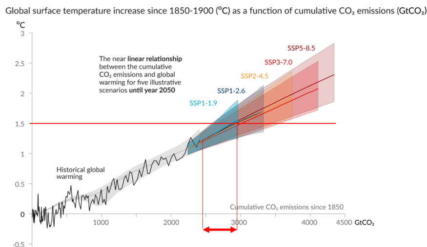
Abb. 9: Temperaturänderung (seit 1850–1900) als nahezu lineare Funktion der gesamten globalen CO 2 -Emissionen seit 1850 (IPCC AR6 (SPM), Fig. SPM.10) (Grafik: https://www.ipcc.ch/report/ar6/wg1/ ). Die schwarze Linie zeigt die historischen Daten und die unterschiedliche Farbe gibt die zusätzliche Menge an CO 2 -Emissionen und die daraus resultierenden Temperaturerhöhungen für die jeweiligen Szenarien für die nächsten 30 Jahre an. Die Schattierungen stellen die entsprechenden Unsicherheitsbereiche dar.
