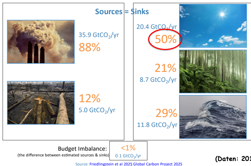
Abb. 3: Quellen (sources) und Senken (sinks) des anthropogen emittierten CO 2 im Erdsystem (Ozean, Biosphäre, Atmosphäre) in Gt CO 2 pro Jahr (1 Gigatonne = 1 Milliarde Tonnen = 10 12 kg). (Grafik: Friedlingstein et al., 2025)
